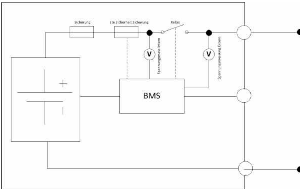
Abbildung 4-35 Blockschaltbild BMZ ESS Slave Batterie
