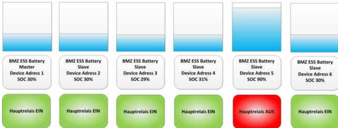
Abbildung 4-37 Darstellung Beispiel 2 unterschiedliche SOC bei parallel geschalteten BMZ ESS Batterien
