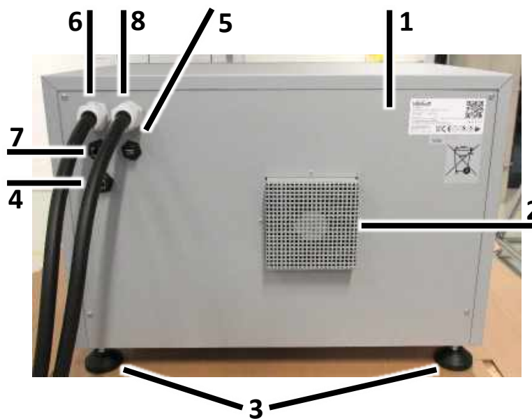
Abbildung 2-5 Batteriespeichersystem, Rückansicht
