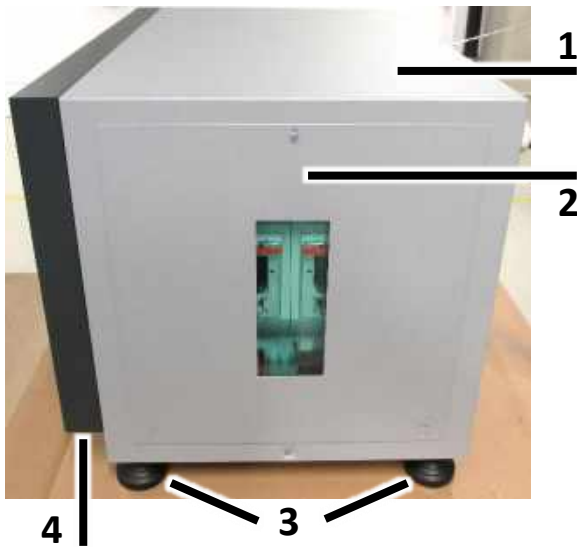
Abbildung 2-3 Batteriespeichersystem, Seitenansicht
