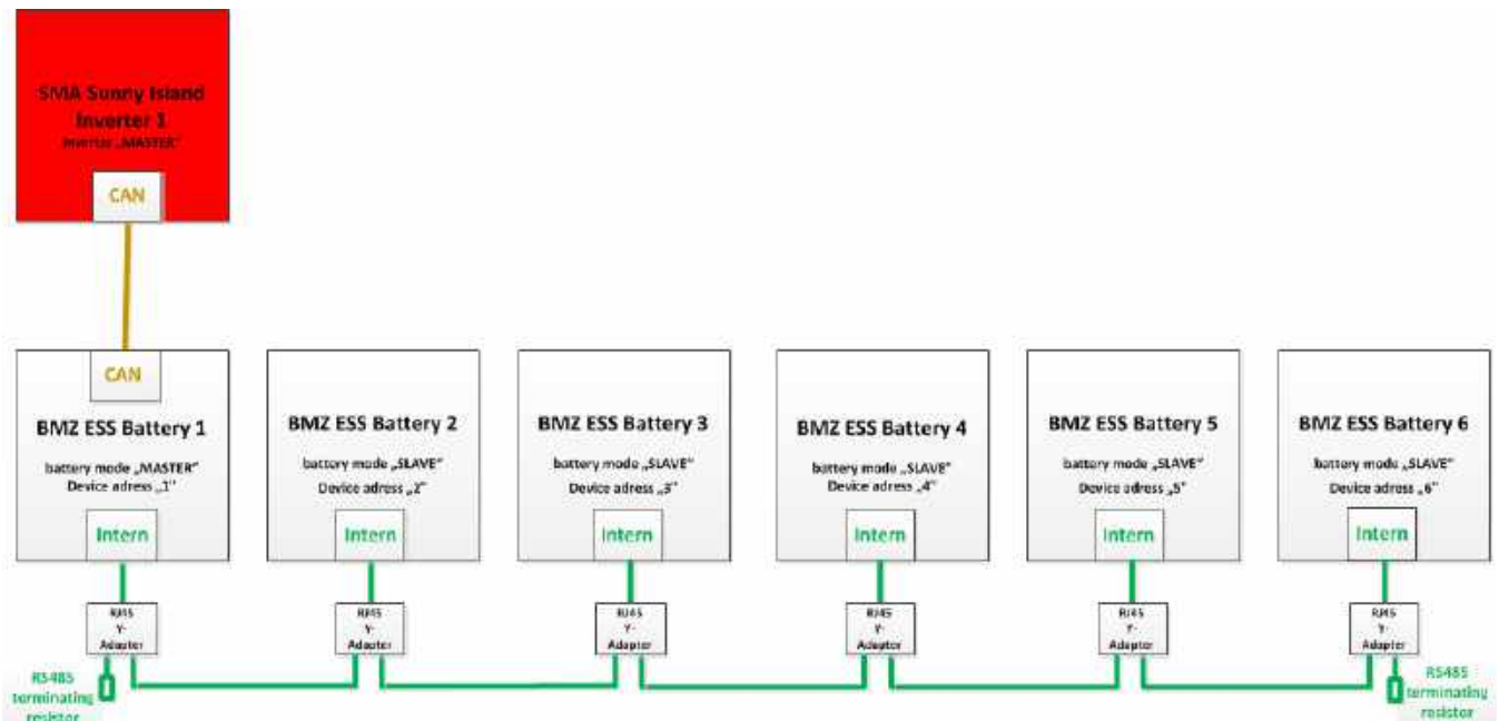
Abbildung 4-10 Kommunikation Verkabelung, Parallelschaltung ESS
