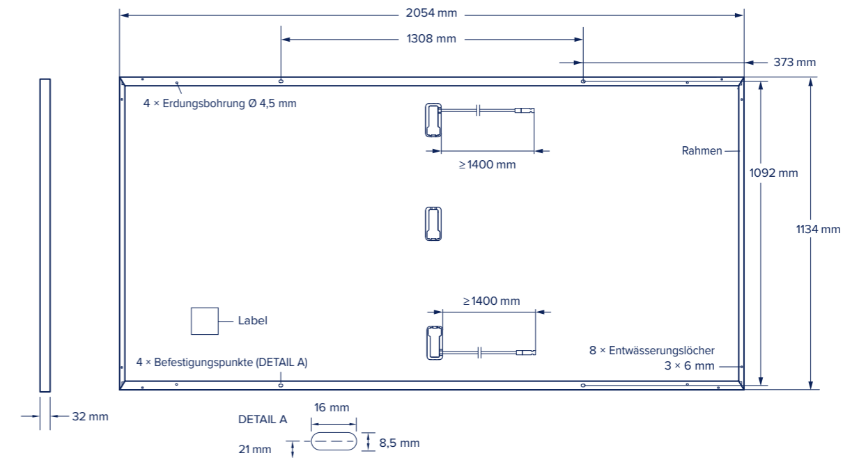
Abb. 1: Außenmaße und Komponenten für Q.PEAK DUO ML-G11.2.
